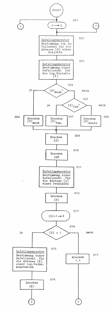
Flußdiagramm für ein Programm der Rechenanlage Zuse Z 22 Abb. 1
